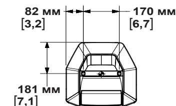
Вид сверху
