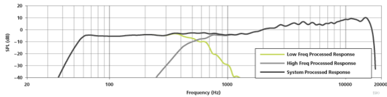
Представлены результаты измерений модуля RM5510; результаты измерений других модулей с вертикальной диаграммой направленности 10°: аналогичные
